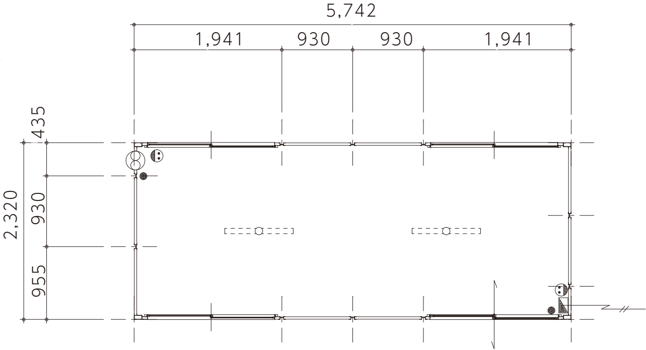
平面図 1:50
