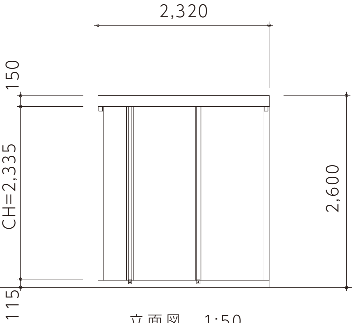
立面図 1:50
