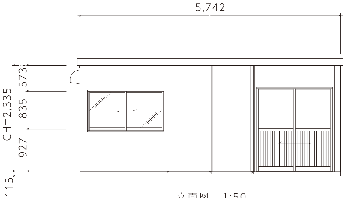
立面図 1:50
